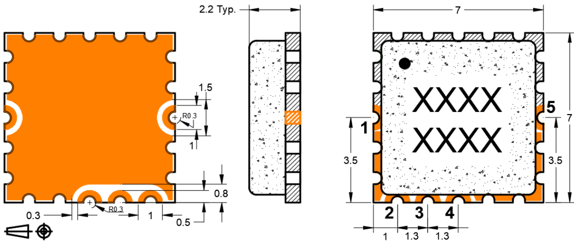
引脚功能
