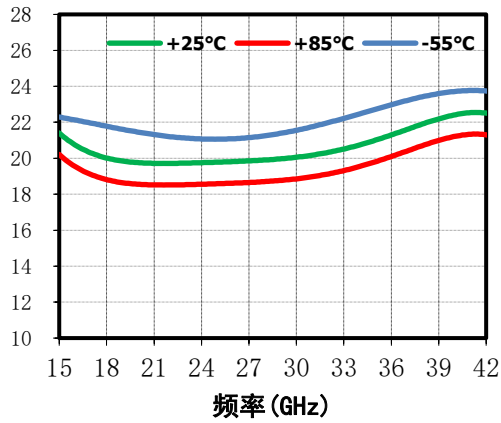
增益(dB) vs. 温度
