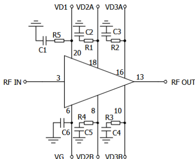
应用电路图
